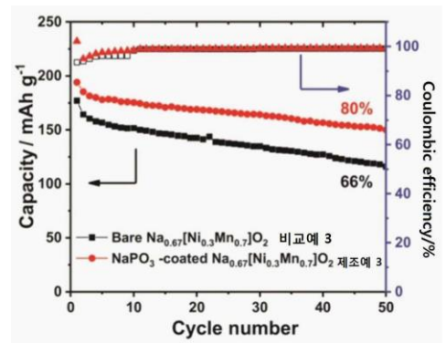
< \text{NaPO}_3 코팅된 양극 활물질의 수명특성 >
