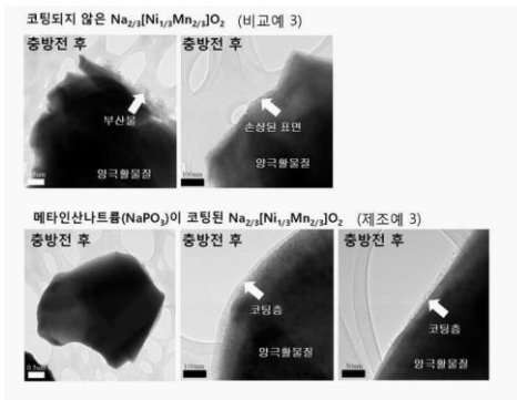
< \text{NaPO}_3 코팅된 양극 활물질의 50 사이클 충방전 후 표면 분석 >
